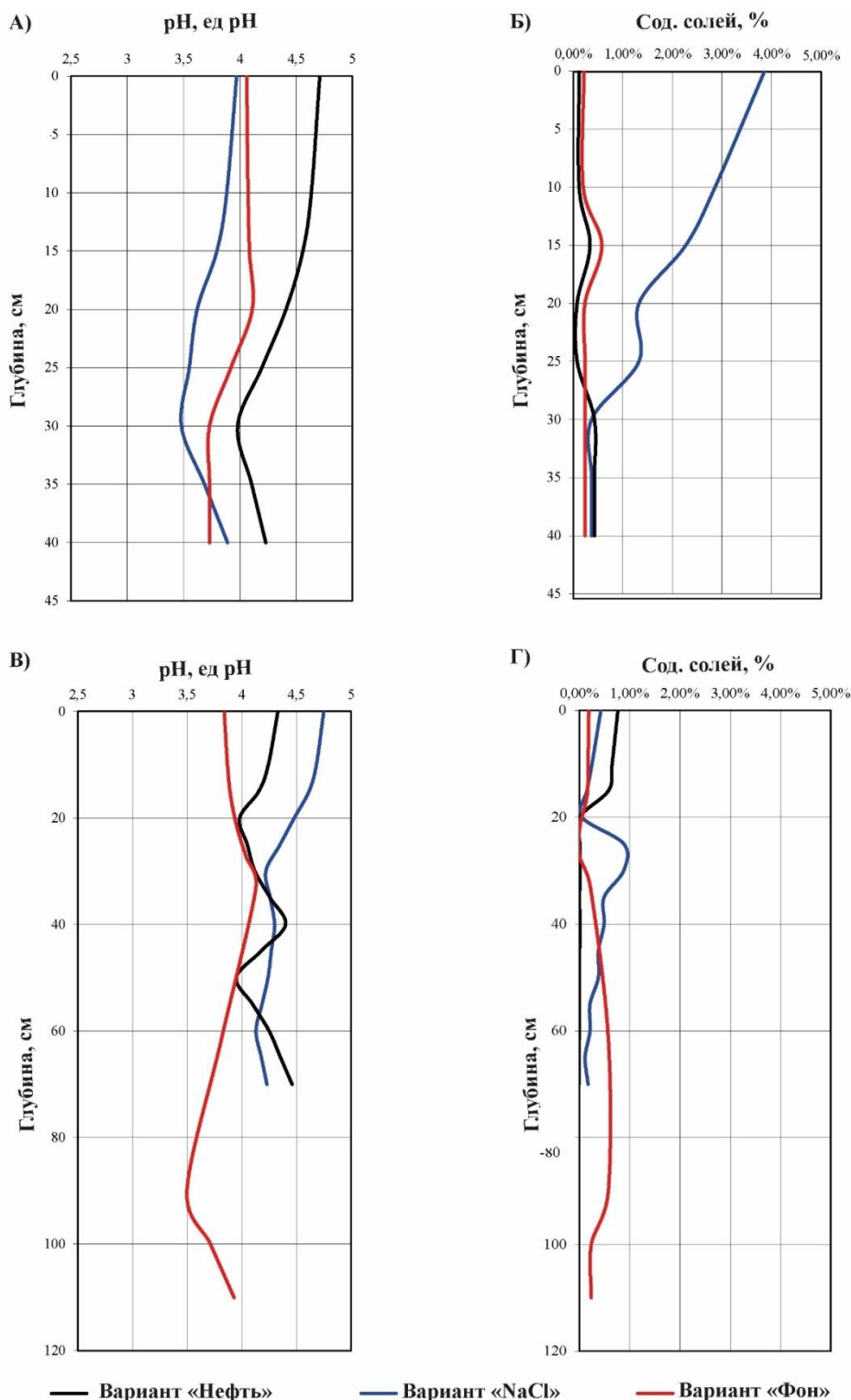
Рис. 4. Динамика изменения по почвенному профилю кислотности pH в ед. pH (А, В) и содержание солей в % (Б, Г): А, Б – для торфяных болотных верховых почв рямовых болот; В, Г – торфяно-подзолисто-глеевых почв (в фоновом состоянии – вариант «Фон»; при загрязнении хлоридно-натриевым раствором – вариант «NaCl», нефтью – вариант «Нефть») Fig. 4. Dynamics of change in soil profile of pH acidity in pH (А, С) and salt content in % (Б, D): А, В – fibric histosols; C, D – histy-gleyic albeluvisols (background state – "Fon" – red; contaminated with chloride-sodium solution – "NaCl" – blue and contaminated with oil – "Oil" – black)
