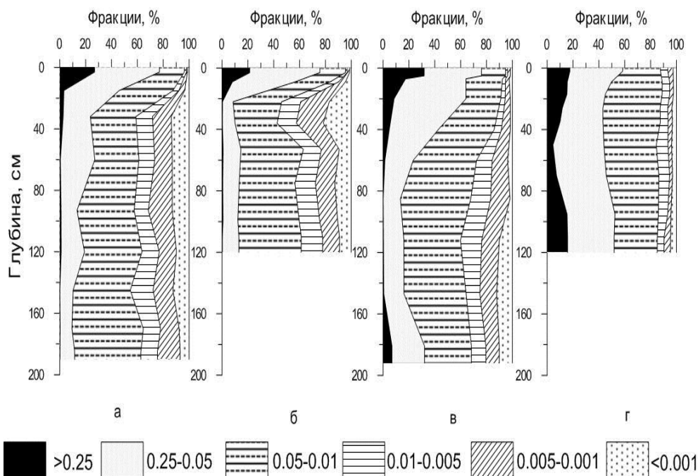
Рис. 5. Профильное распределение микроагрегатов в исследуемых почвах, разрезы: a – 3-011;
