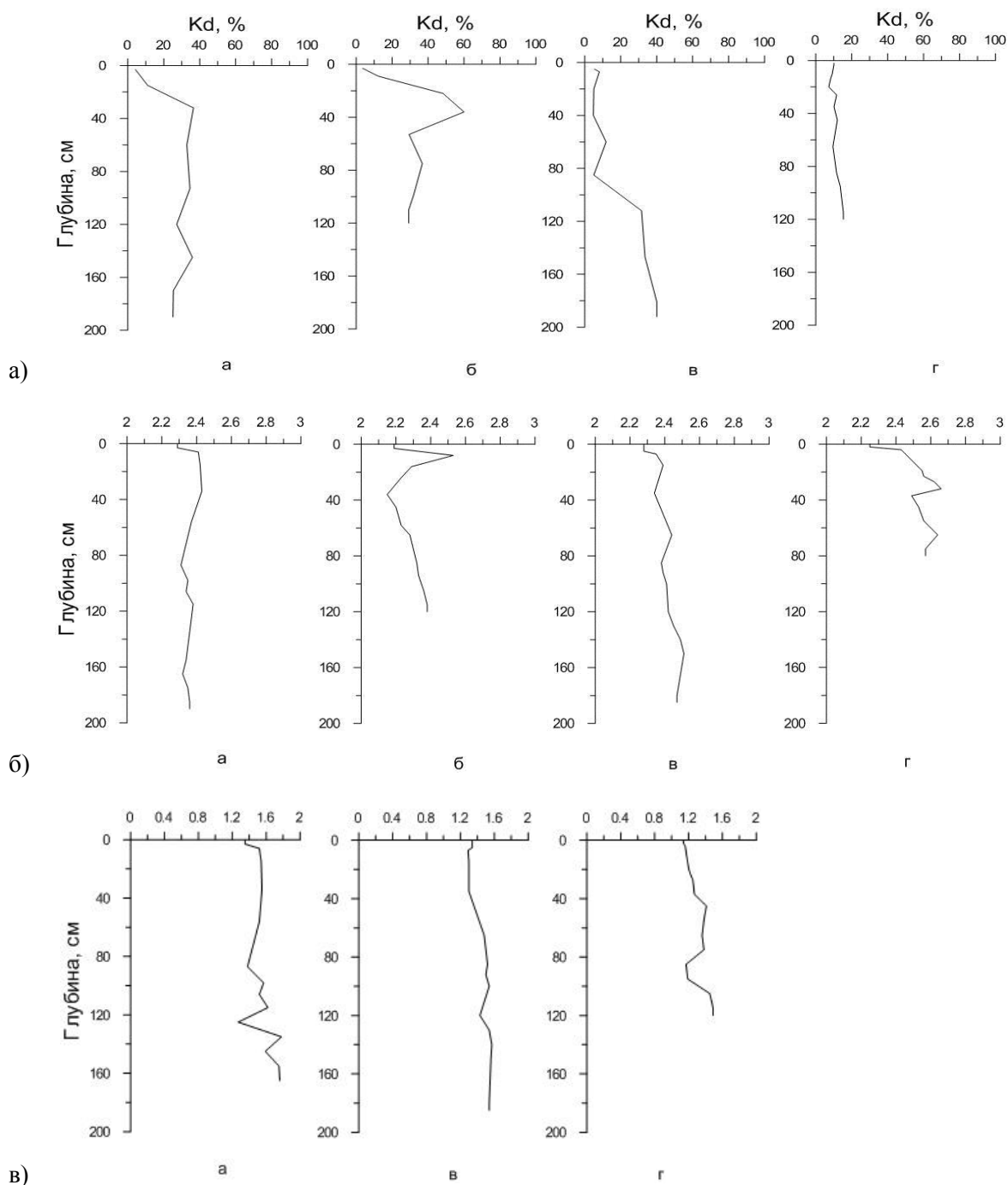
Рис. 6. Некоторые физические характеристики изученных почв: а – коэффициент дисперсности; б – плотность твердой фазы; в – плотность сложения. Обозначение разрезов: а – 3-011; б – 32-011; в – 4-011; г – 1-012
