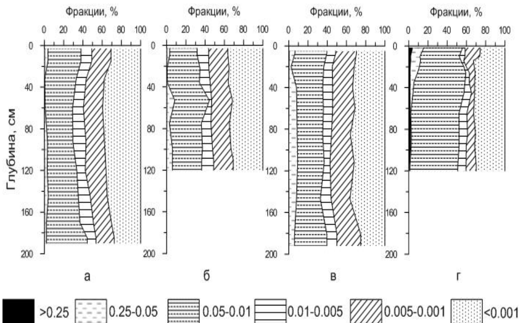
Рис. 4. Гранулометрический состав современной и древней частей почв, разрезы:
