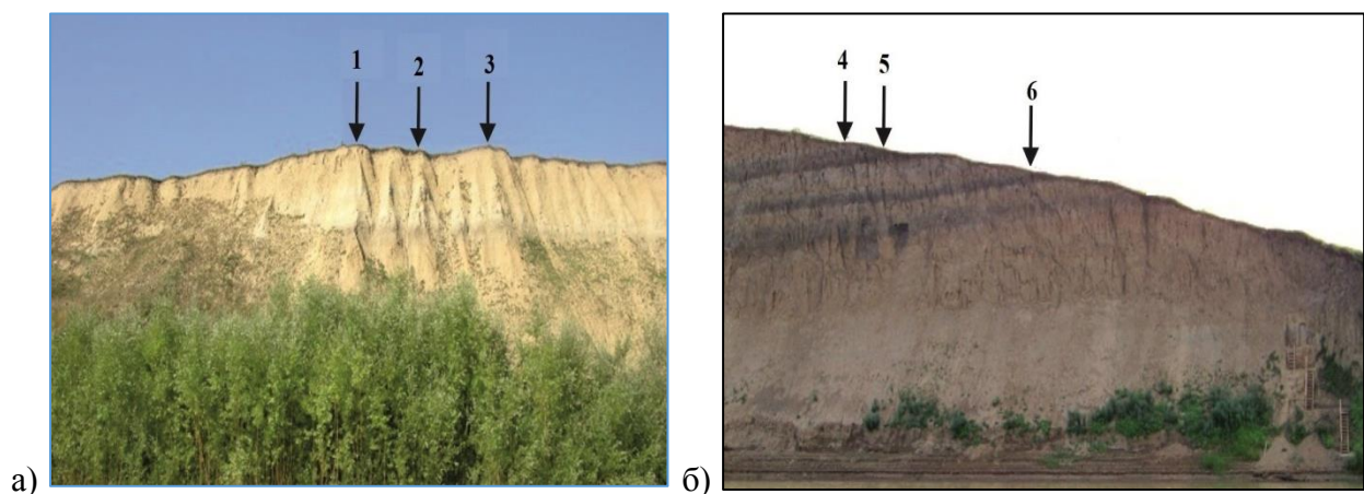
Рис. 2. Расположение почв: а – без признаков древнего педогенеза (разрезы: 1 – 1-06; 2 – 1-010Д; 3 – 1-012); б – с признаками древнего педогенеза (разрезы: 4 – 3-011; 5 – 32-011; 6 – 4-011) Fig. 2. Location of soils: а – without features of ancient pedogenesis (sections: 1 – 1-06; 2 – 1-010Д; 3 – 1-012); б – with features of ancient pedogenesis (sections: 4 – 3-011; 5 – 32-011; 6 – 4-011)
