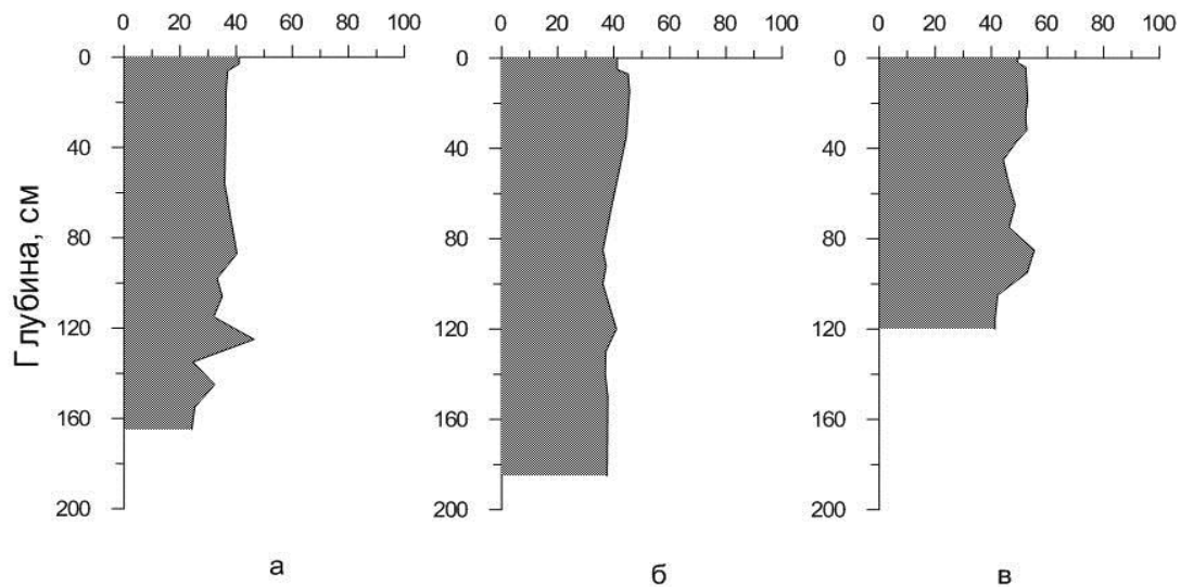
Рис. 7. Общая порозность в исследуемых почвах. Обозначение разрезов: а – 3-011; б – 4-011; в – 1-012
