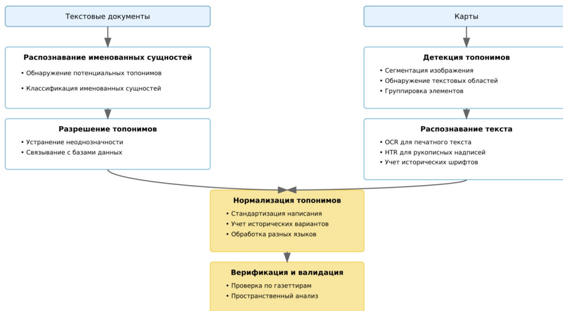
Рис. 1. Схема автоматической обработки топонимов из географических карт и текстов Fig. 1. Diagram of automatic processing of toponyms from geographical maps and texts
