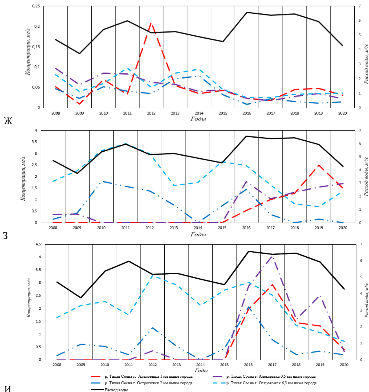
Рис. 2. Динамика гидрохимических показателей на постах наблюдений: Ж – содержание железа; 3 – содержание меди; И – содержание цинка (окончание)
