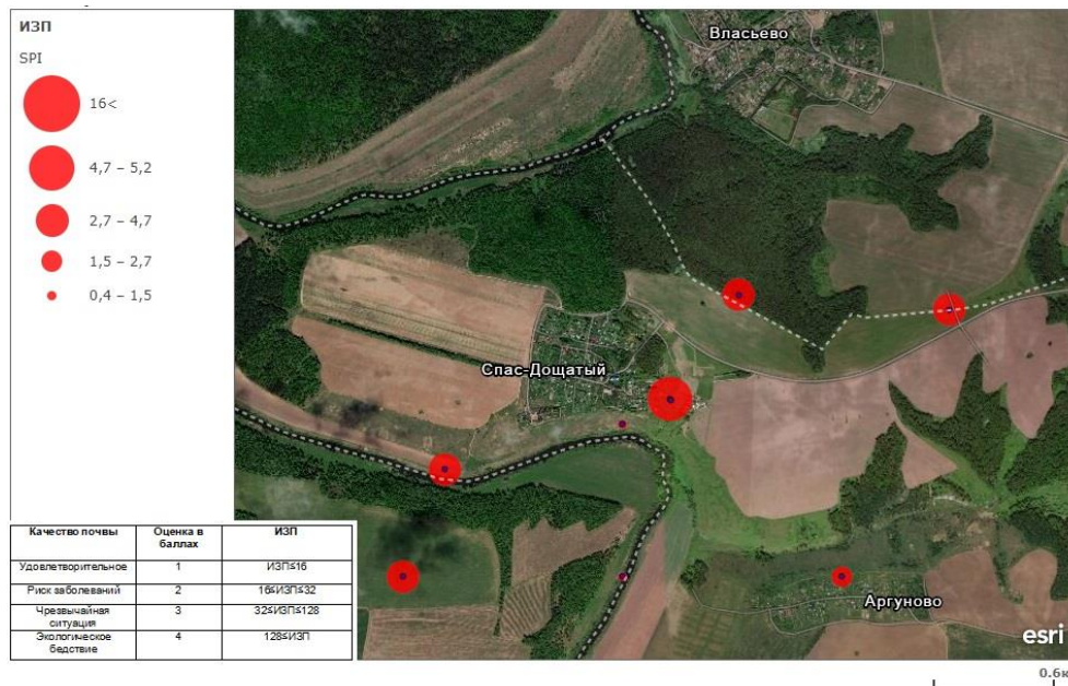
Рис. 2. Классификация качества почвы в зависимости от значений ИЗП (2019 г.)
