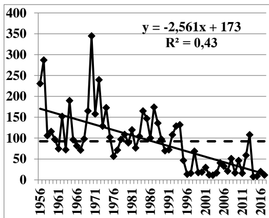
Рис. 3. Экстремумы стока р. Девица – с. Девица: а – максимального; б – минимального Fig. 3. Extremes of runoff r. Devitsa – Devitsa: a – maximum; б – minimum
