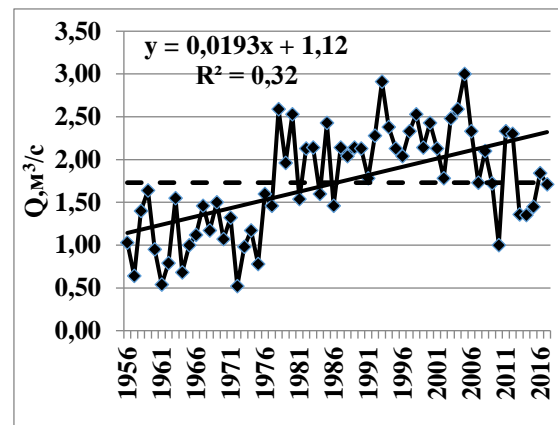
Рис. 3. Экстремумы стока р. Девица – с. Девица: а – максимального; б – минимального Fig. 3. Extremes of runoff r. Devitsa – Devitsa: a – maximum; б – minimum
